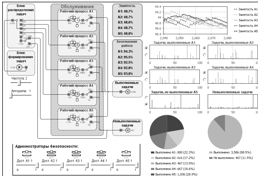
Рис. 2. Модель АСА КСПД в среде моделирования AnyLogic
